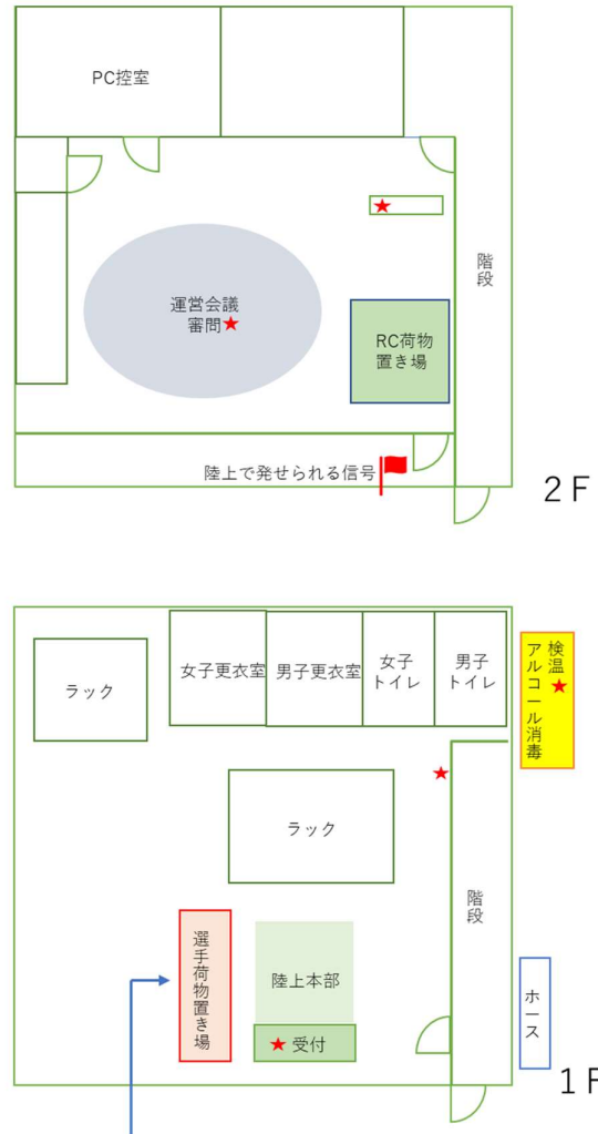
8.2 ハウス 見取り図
